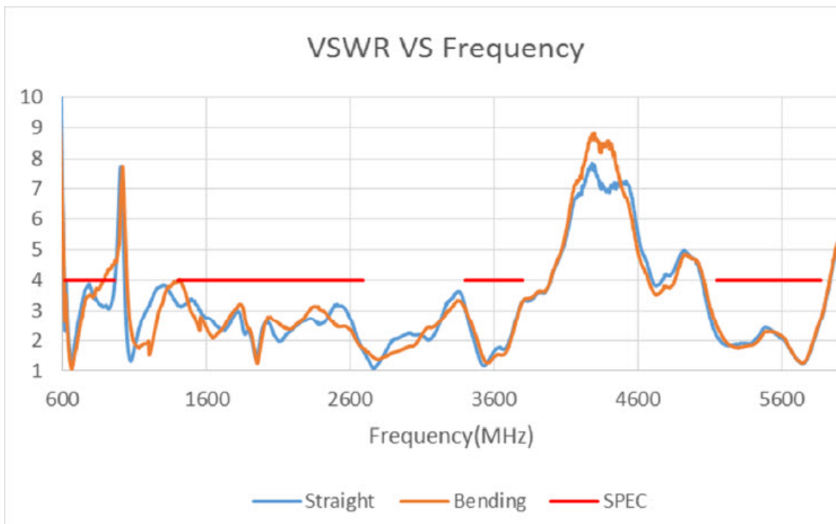
図 3: VSWR と周波数
