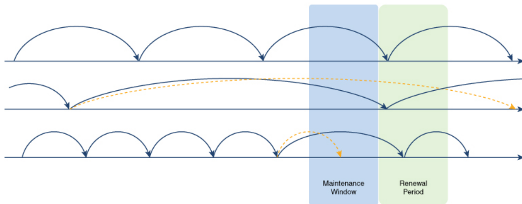
図 1 : Maintenance Window
