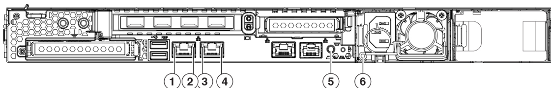
Figura 10: LED del panel posterior y sus estados
