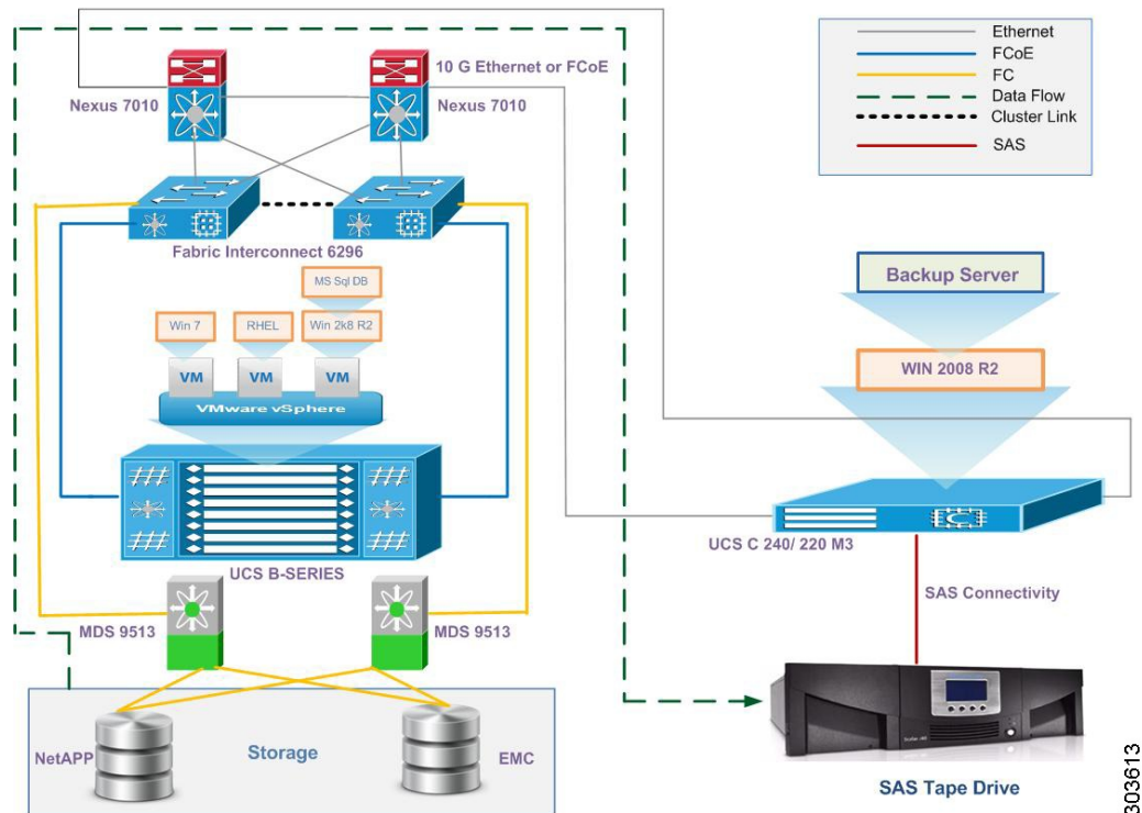
図 1: バックアップテスト SAS 構成 (バックアップサーバをスタンドアロン C シリーズサーバに配置)
