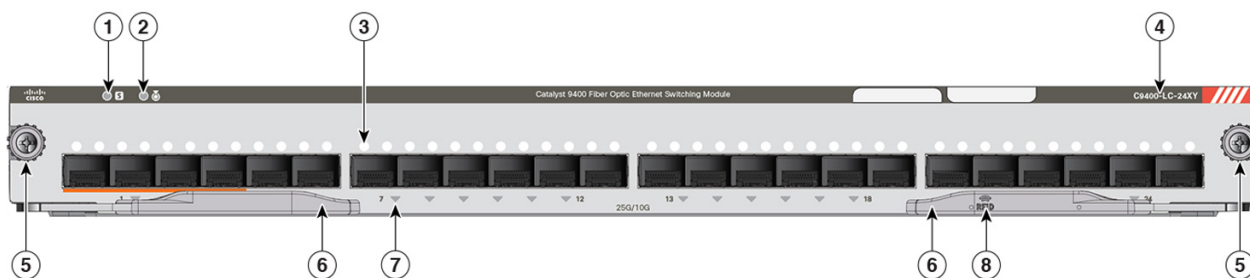
Figura 13: Vista frontale della scheda di linea C9400-LC-24XY
