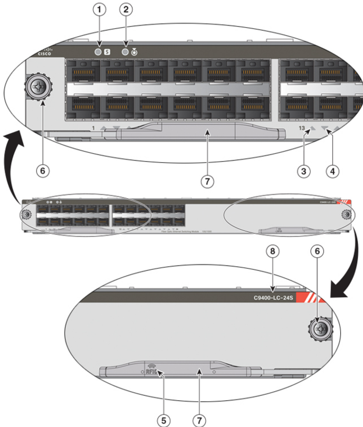
Figura 11: Vista frontale della scheda di linea C9400-LC-24S
