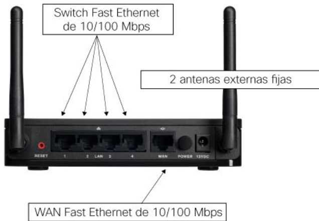
Figura 2. Panel posterior del Cisco RV110W – Wireless –N Firewall VPN
