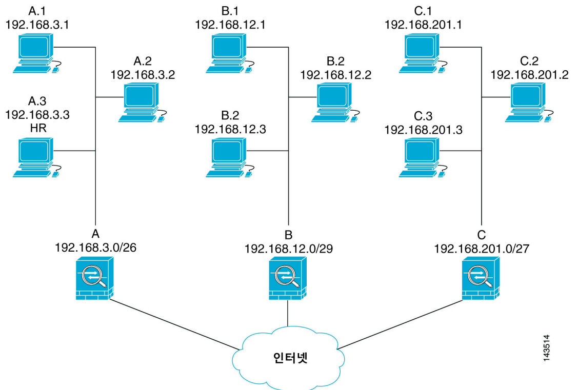
그림 1-3 트래픽의 Permit 및 Deny ACE 효과 (실제 주소)
