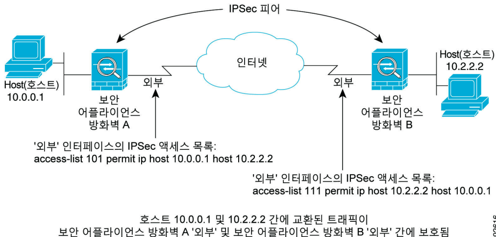
그림 1-4 암호화 ACL을 IPsec에 적용하는 방법
