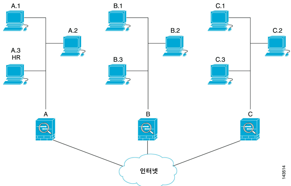
그림 1-1 트래픽의 Permit 및 Deny ACE 효과(개념적 주소)
