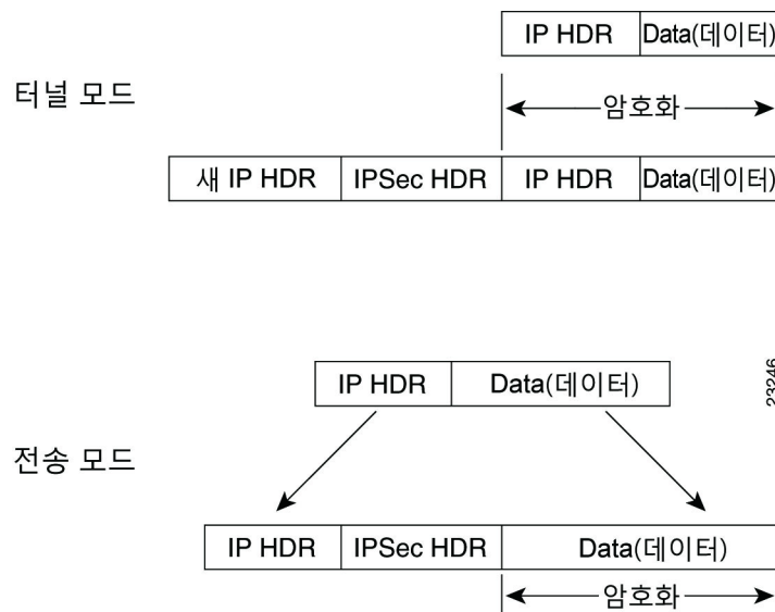
그림 2-1 터널 모드와 전송 모드의 IPsec
