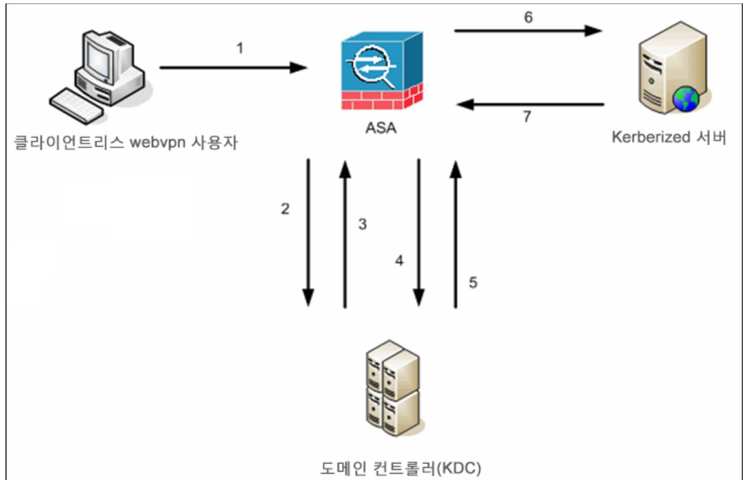
그림 15-1 KCD 프로세스
